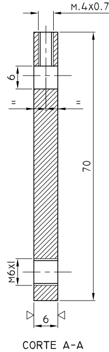
CORTE A-A
